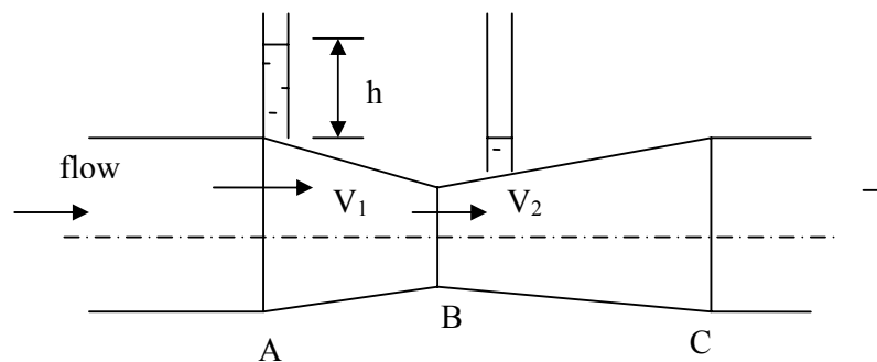
Fig. A venturi meter
