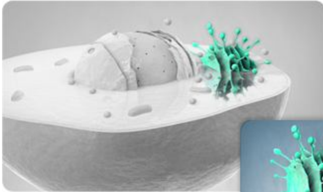
Golgi apparatus
