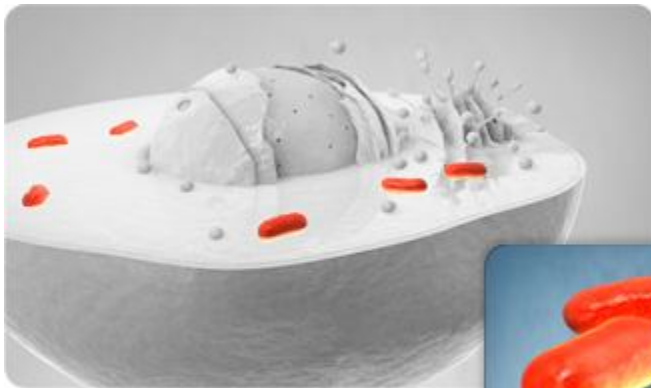
Mitochondria
